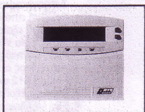
NX-148GR LCD alphanumeric με φωτιζόμενα πλήκτρα, πορτάκι και Ελληνικούς / Αγγλικούς χαρακτήρες. Διαστάσεις: Π 15.8 x Υ 13.5 x Β 3cm
